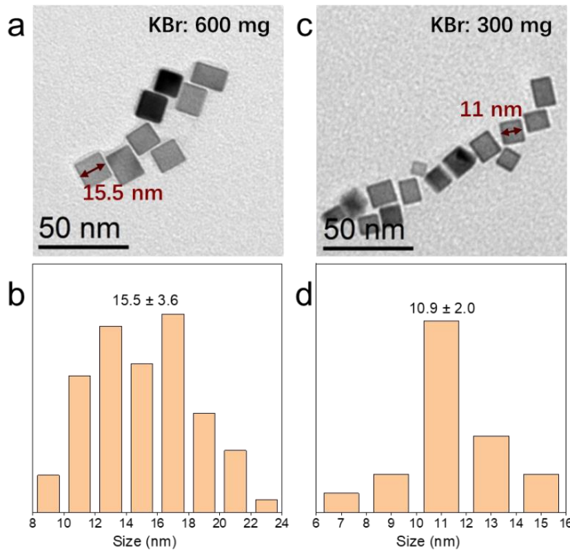
钯纳米立方颗粒的 TEM 图与粒径分布
